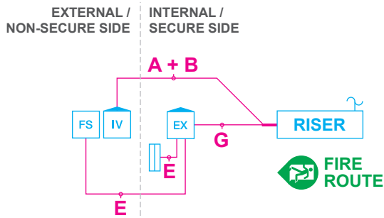
T N° 070/1 IPVIEW + Fireman Switch
