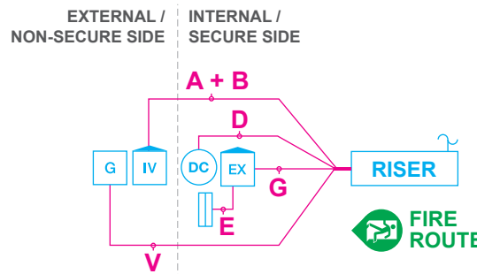
T N° 071/1A IPVIEW + DC + GERDA
