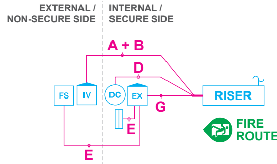
T N° 070/1A IPVIEW + DC + Fireman Switch
