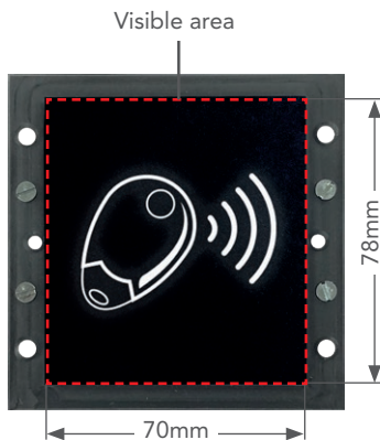
LPMRS-XNA Module
